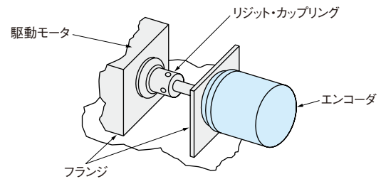
図-8 リジッドなカップリング (悪い例)
