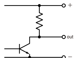
電圧出力
