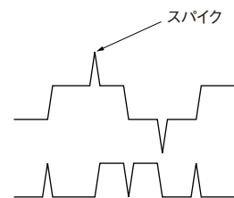
図-3 スパイク波形
